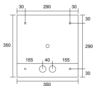
Bohrabstände W1 Drilling distances W1
