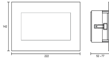
KI Einbau / recessed
